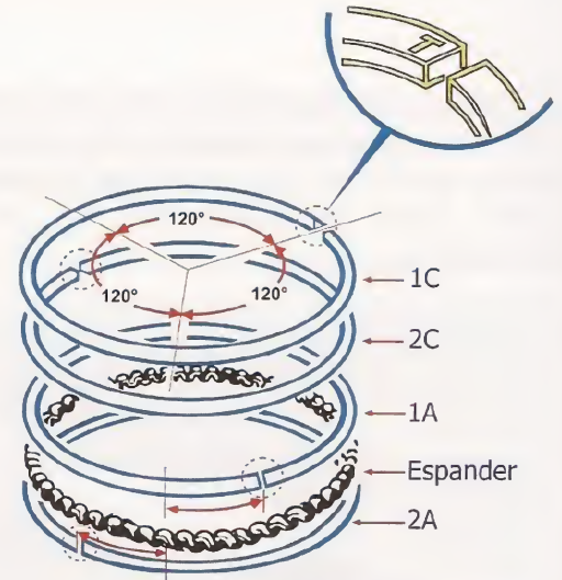
Posición de anillos a 120°
